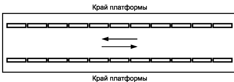
Рисунок А.4 — Форма рифления — одноэлементная тактильная полоса с плоской вершиной (щучлиния), используемая для обустройства протяженных предупреждающих ТНУ вдоль края платформ различного назначения
